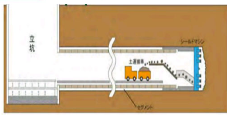
シールド工法概要図
