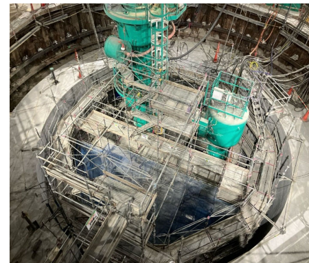
立坑内【現状】
