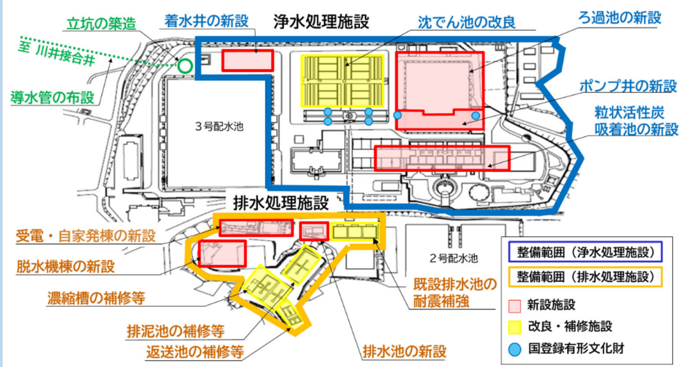
図 2 西谷浄水場の整備範囲
