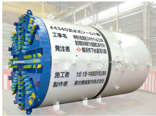
シールドマシン(内径3750mm)
