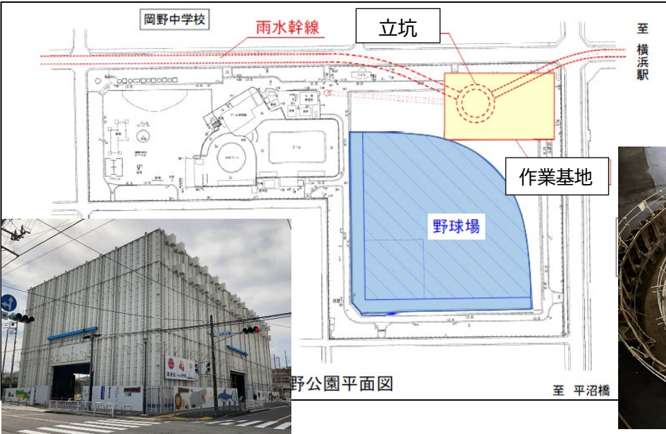
作業基地外観(防音ハウス設置)
