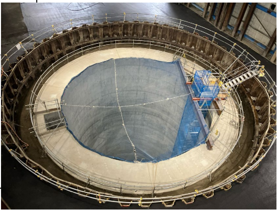
完成した特殊人孔(立坑)の様子
